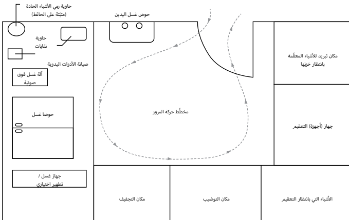
الرسم 1: تخطيط مقترح لمكان التعقيم (AS/NZS 4815-2006)
