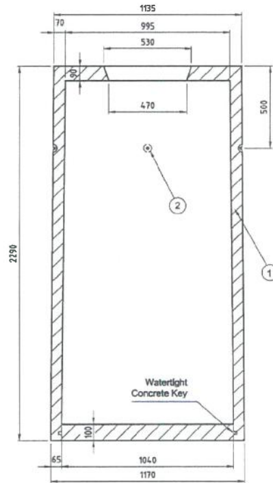
SECTION A-A
