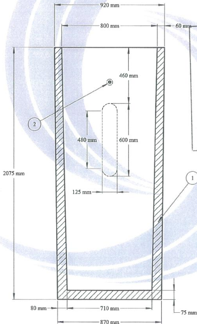
SECTION A-A
